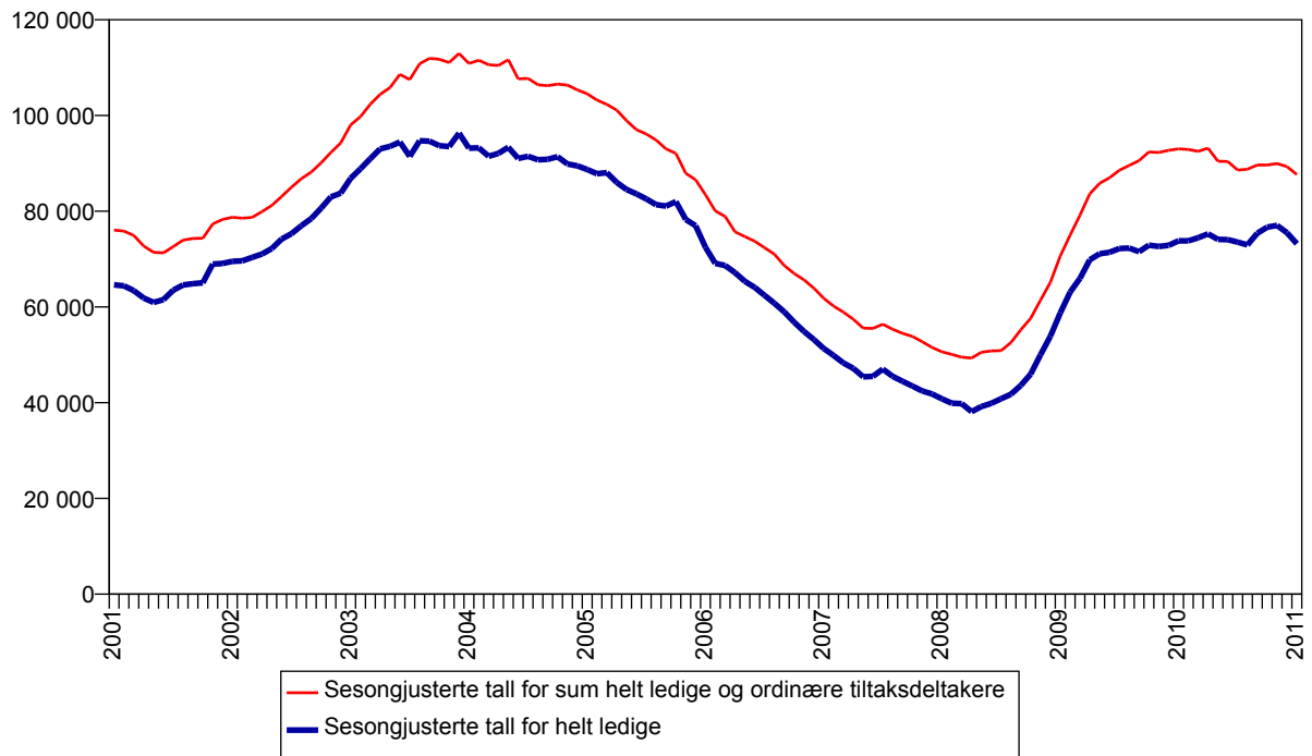
Figur 1: Sesongjusterte tall for helt ledige og summen av helt ledige og ordinære tiltaksdeltakere. 2001 - januar 2011
