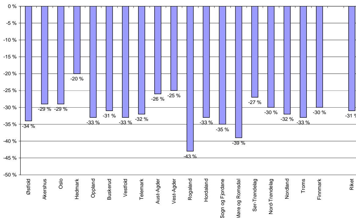
Figur 6. Prosentvis endring i antall registrerte ledige fordelt på fylke. Desember 2005 – desember 2006.
