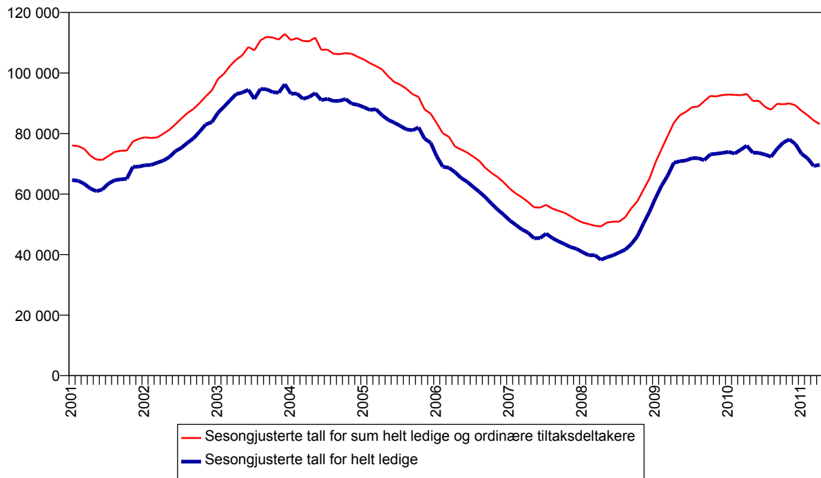
Figur 1: Sesongjusterte tall for helt ledige og summen av helt ledige og ordinære tiltaksdeltakere. 2001 - april 2011
